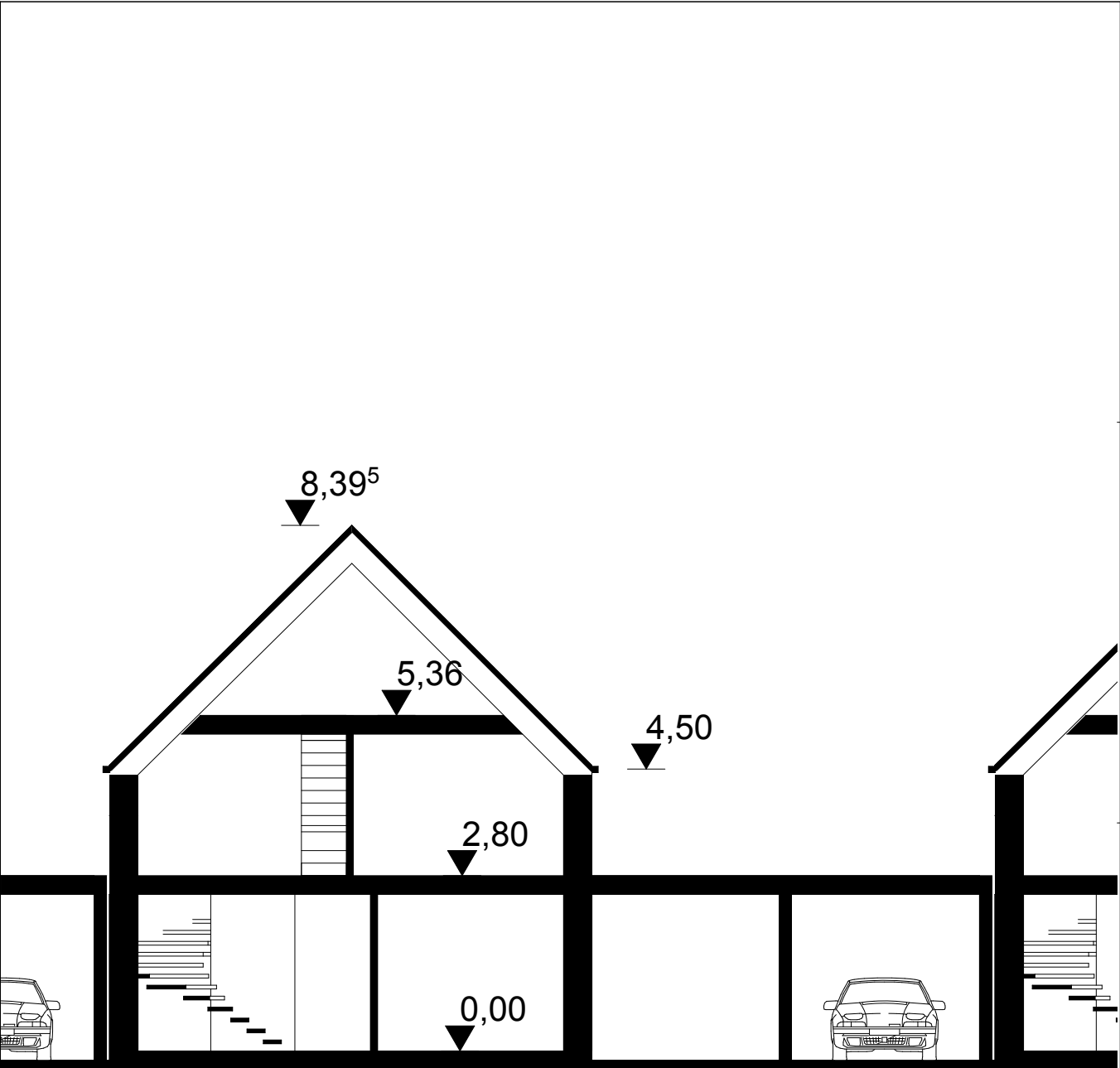
Schnitt
