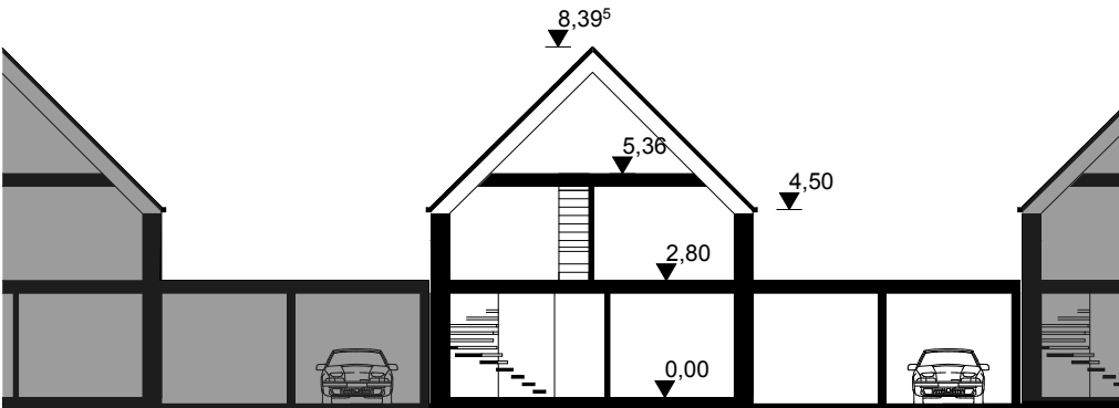
SCHNITT
